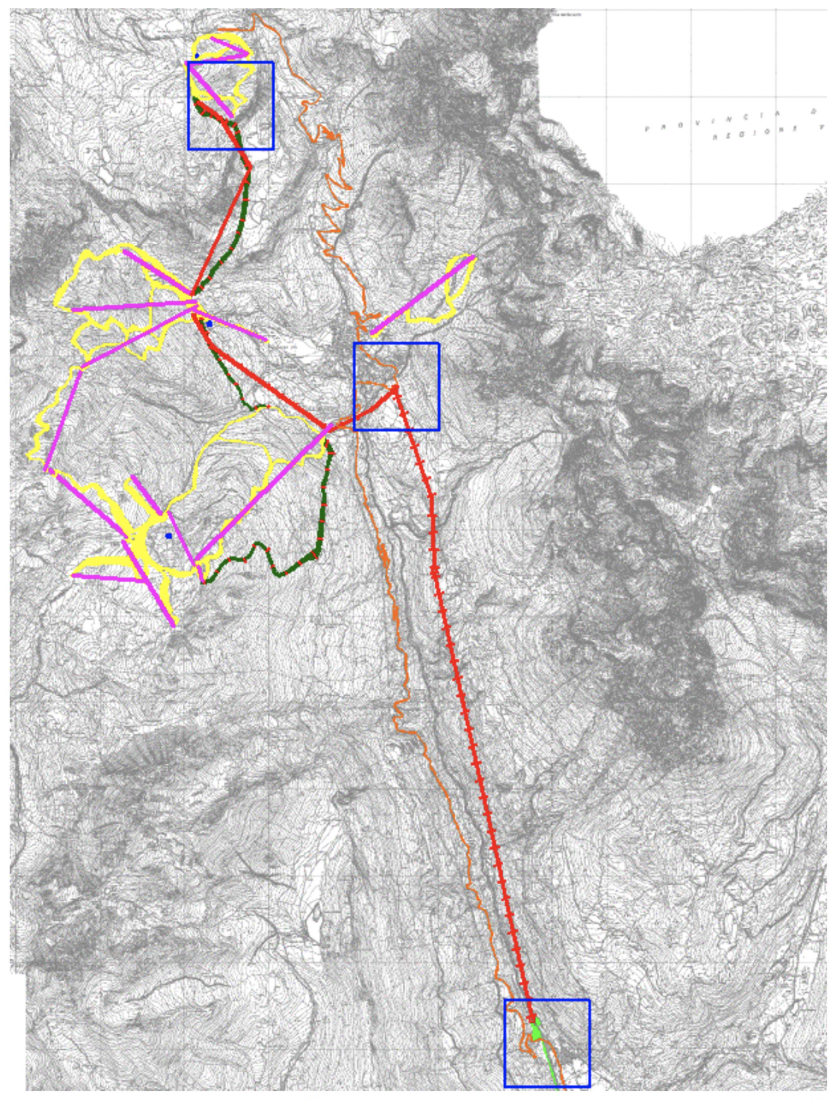
Tracciato di progetto collegamento Siror – S.Martino-Passo Rolle
