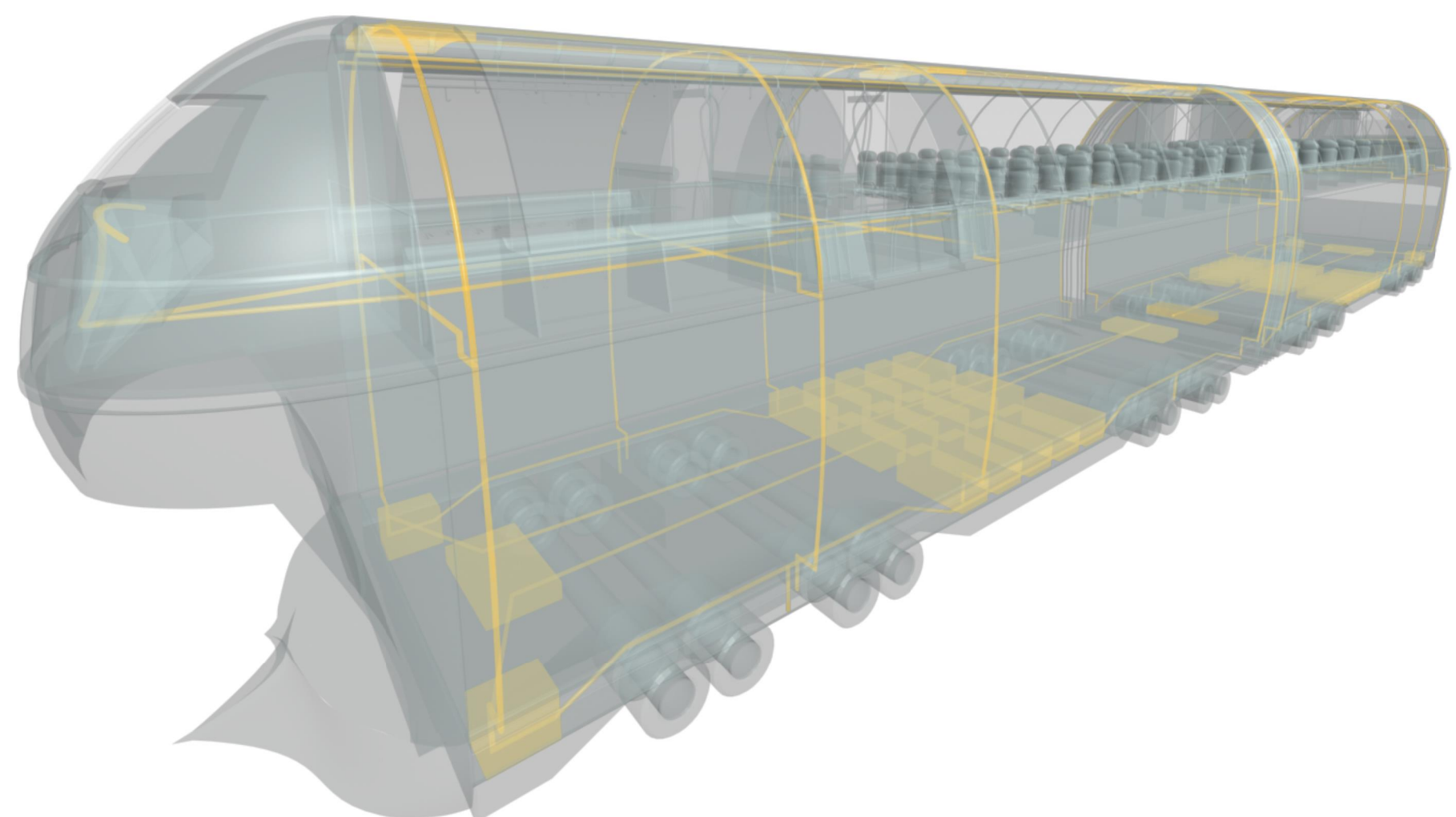
Disposizione interna batterie – full cell
